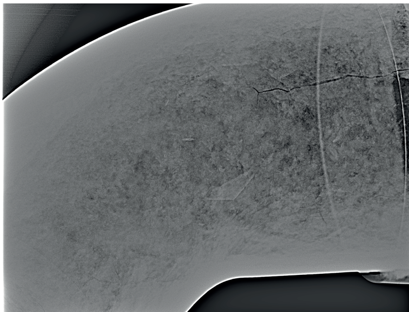
Kuva: Valurautaisen jätevesiviemärin läpivalaisukuvasta löytyi halkeama ja korroosiota.
